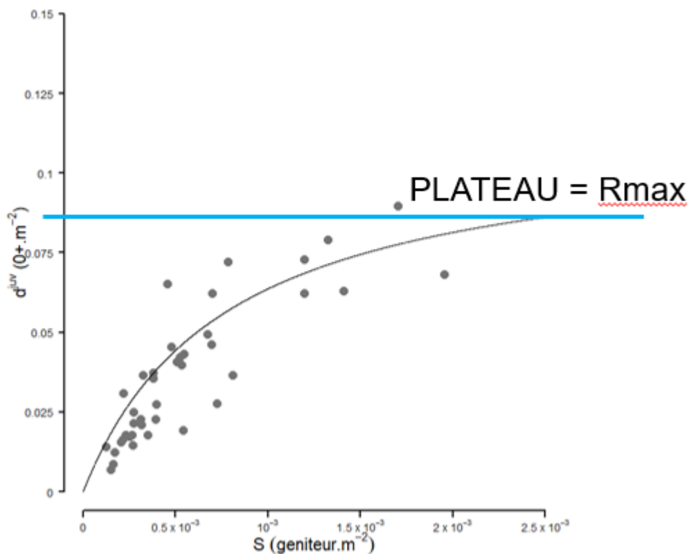
Figure 19 : Courbe de stock recrutement permettant de visualiser la définition de la capacité d'accueil qui correspond au Rmax, c'est à dire à la valeur plateau. On peut ajouter plus de géniteurs dans le milieu, on ne produira pas en moyenne plus de juvéniles (Source : Legrand & Prévost, 2018)
