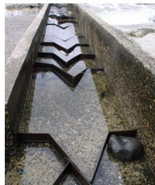
Figure 36 : Passe avec des ralentisseurs dégradés
